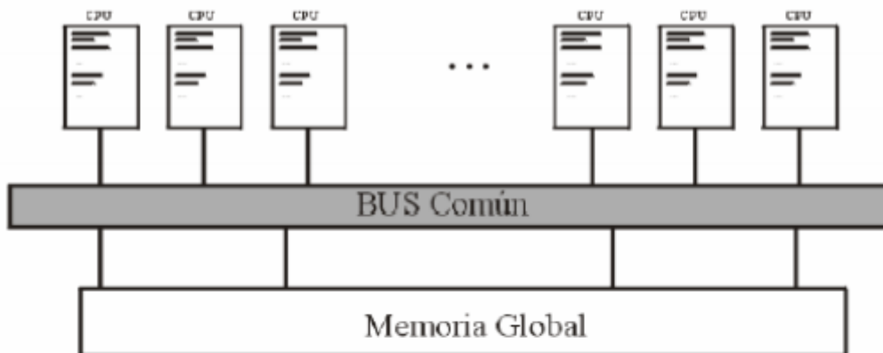
Arquitecturas de memoria compartida
