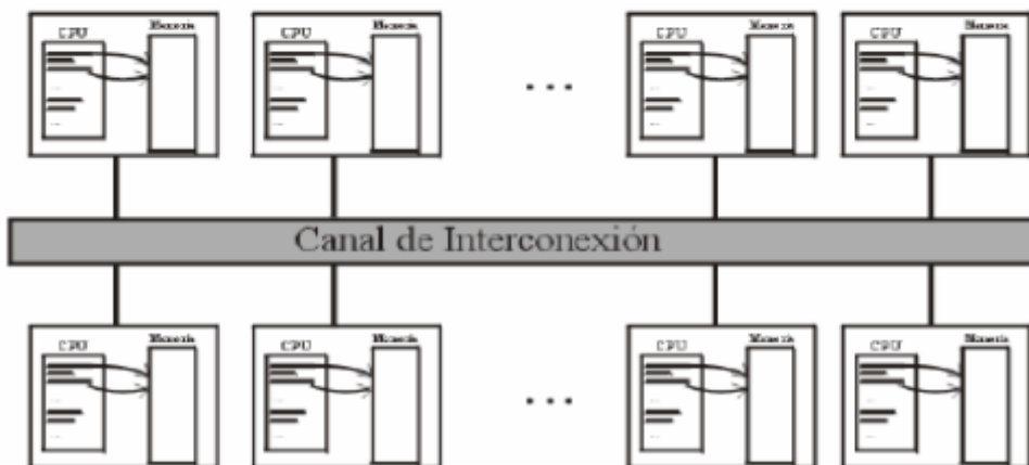
Arquitecturas de memoria distribuida
